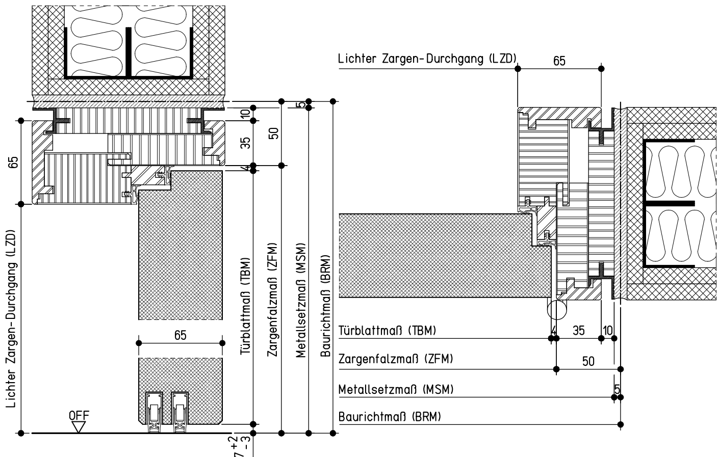
Vertikalschnitt A-A
