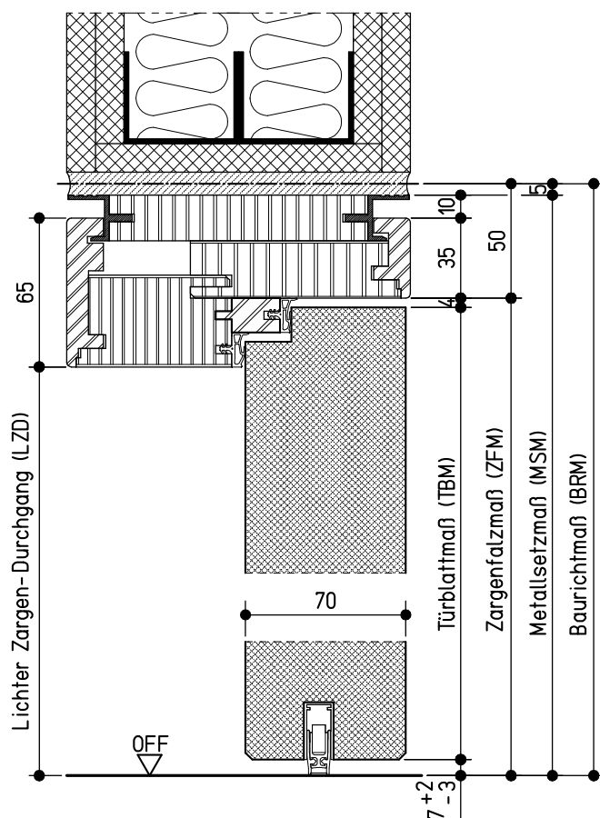
Vertikalschnitt A-A
