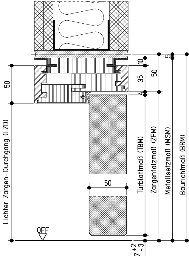
Vertikalschnitt A-A
